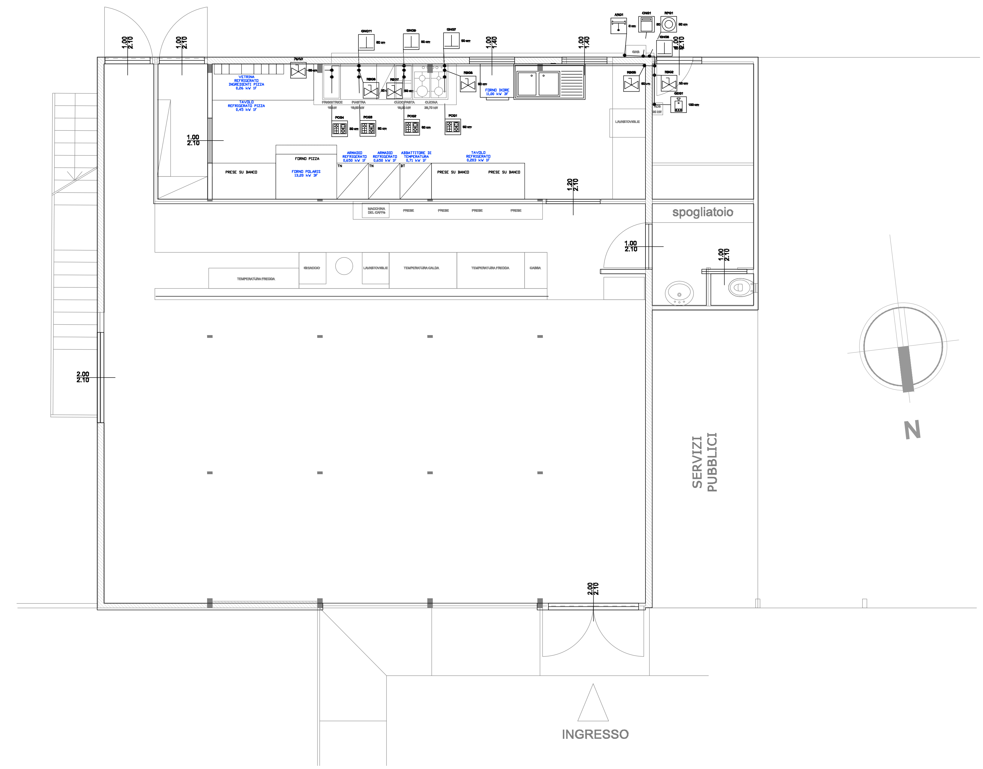
PIANTA SCALA 1:50
